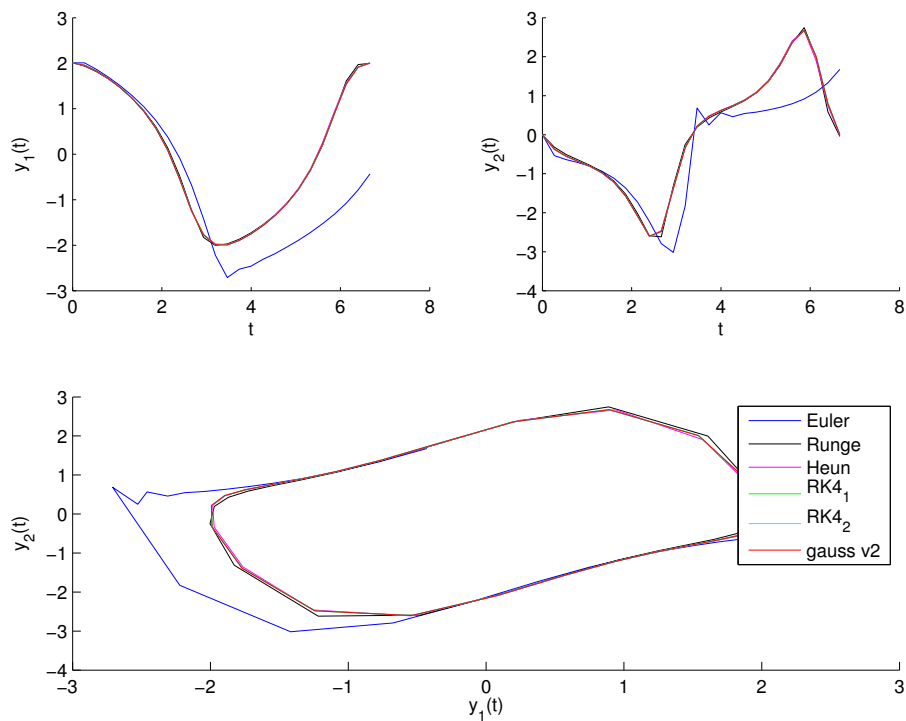
FIGURE 2 – Solution de l'équation de Van der Pol, composante 1 et 2 et plan de phase, pour les schémas de Runge-Kutta avec N = 25 , pour Gauss nb\_itmax = 15 et f\_eps = 1.e-12 .
