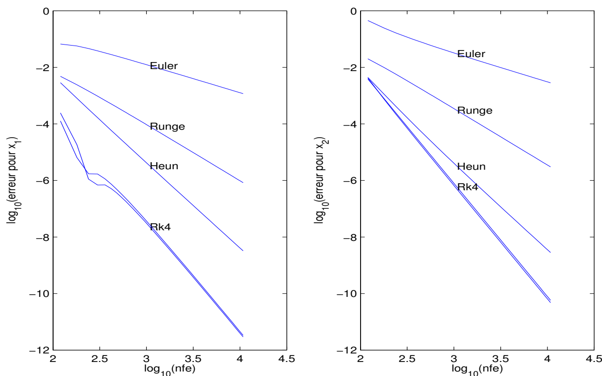
FIGURE 1 – Erreur globale en fonction du nombre d'évaluations, E. Hairer, S.P. Nørsett and G. Wanner, Tome I, page 140, \log_{10}(\text{err}) = C_1 - p \log_{10}(\text{nfe}) .
